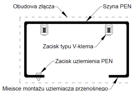
Rys. 1. Przykładowy profil szyny PEN.
