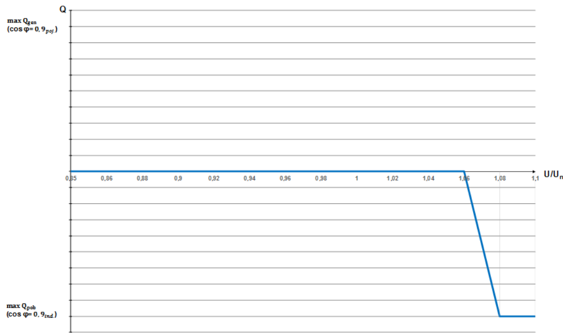
Rys. 4. Charakterystyka sterowania mocą bierną w funkcji napięcia dla mikroinstalacji podłączonych jednofazowo, wymagana przez PGE Dystrybucja S.A.
